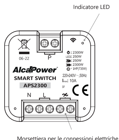
Morsettiera per le connessioni elettriche
